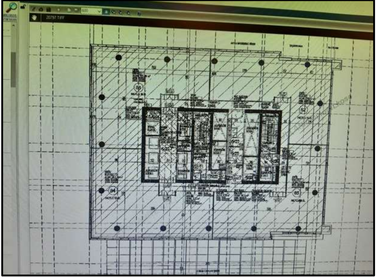
B BLOK TİP KULE KAT PLANI
